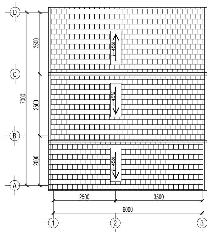
MẶT BẰNG MÁI TL 1/100
