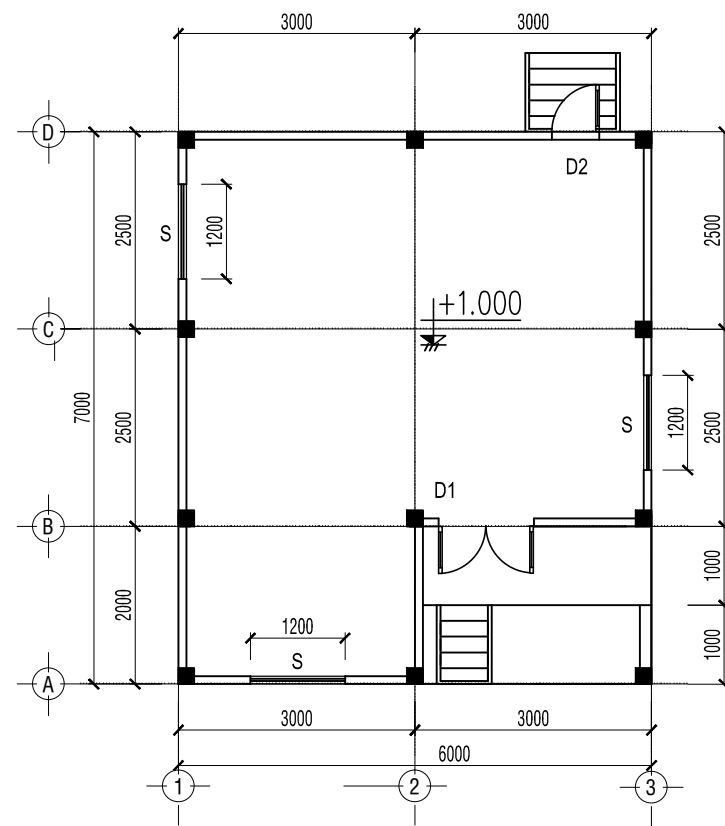
MẶT BẰNG TRỆT TL 1/100
