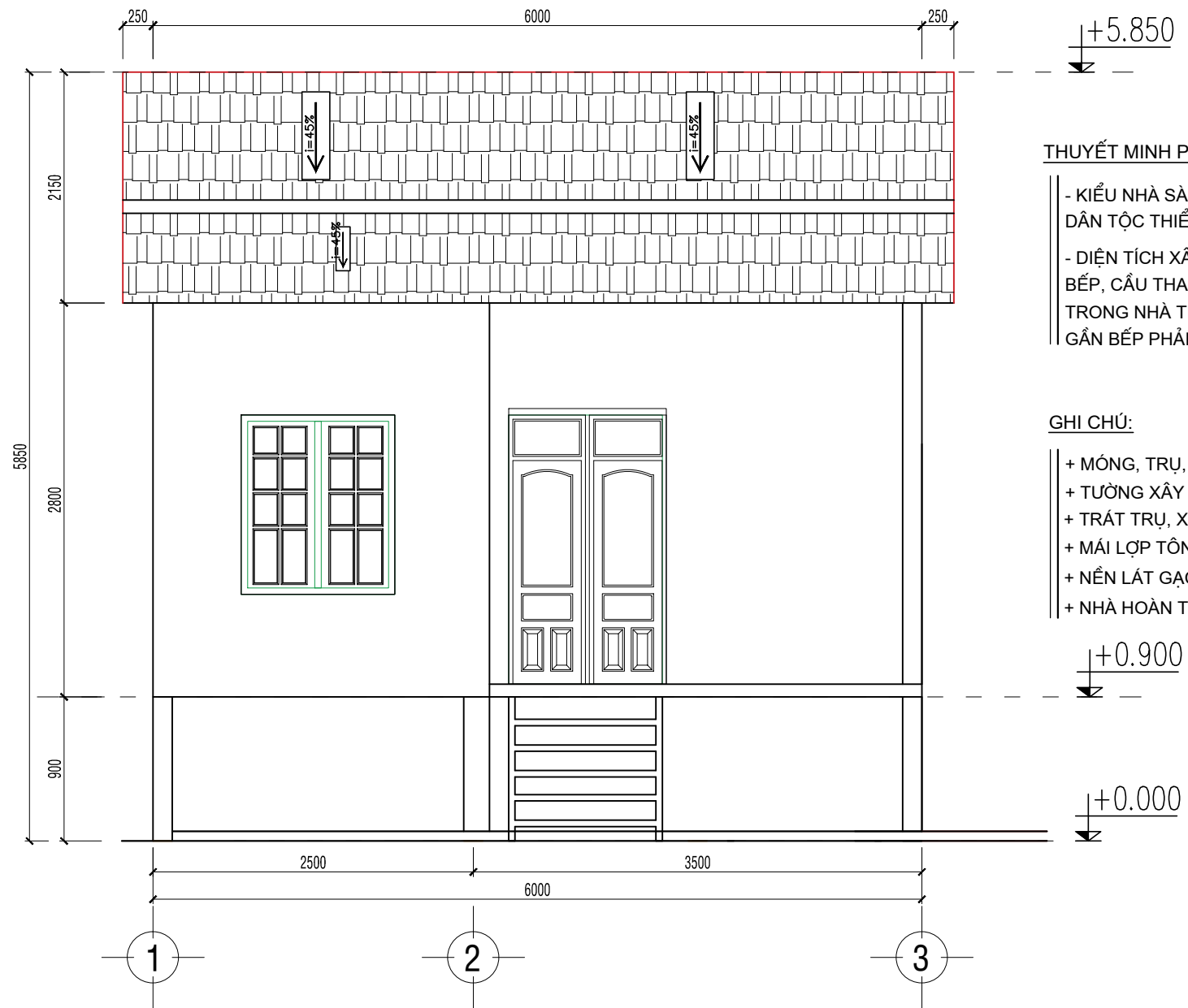
MẶT ĐỨNG TRỰC 1-3 TL 1/50
