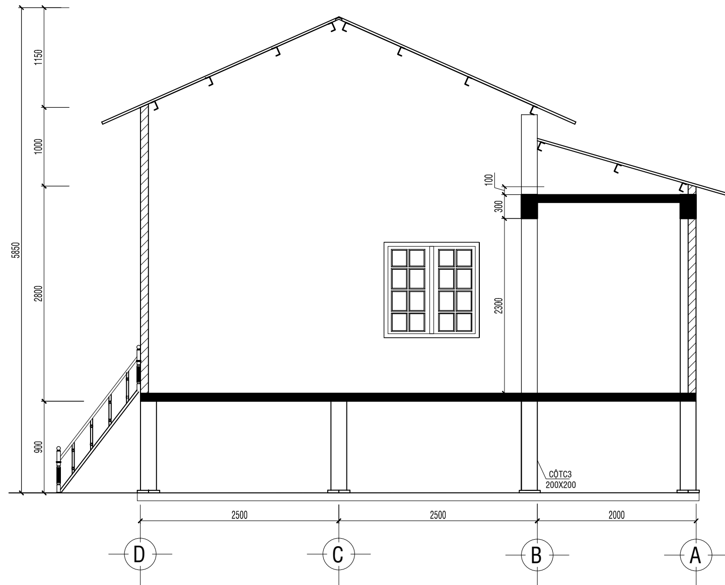
MẶT ĐỨNG TRỤC D-A TL 1/50
