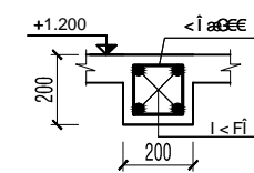
CHI TIẾT DẦM SÀN D1,...D4
