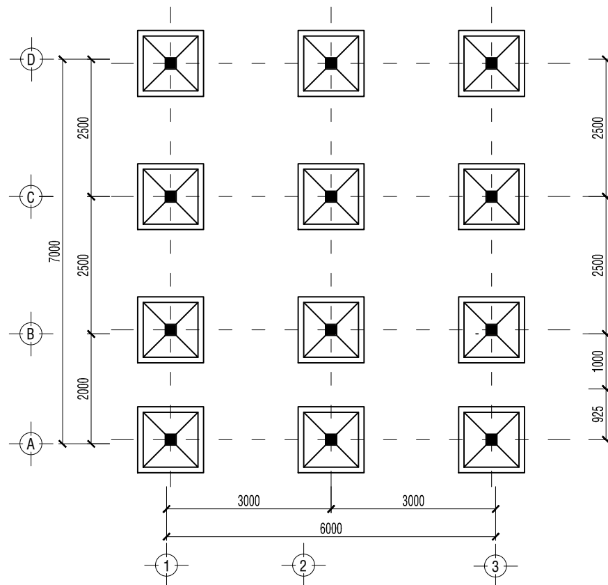
MẶT BẰNG CỘT MÓNG M1C1, TL 1/100
