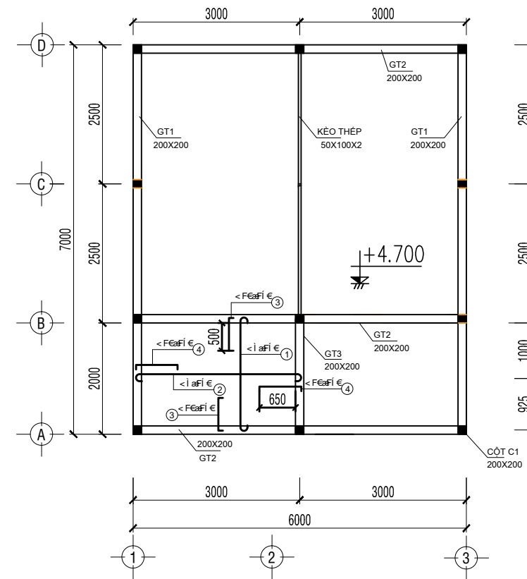
MẶT BẰNG GIẰNG TƯỜNG TL 1/100
