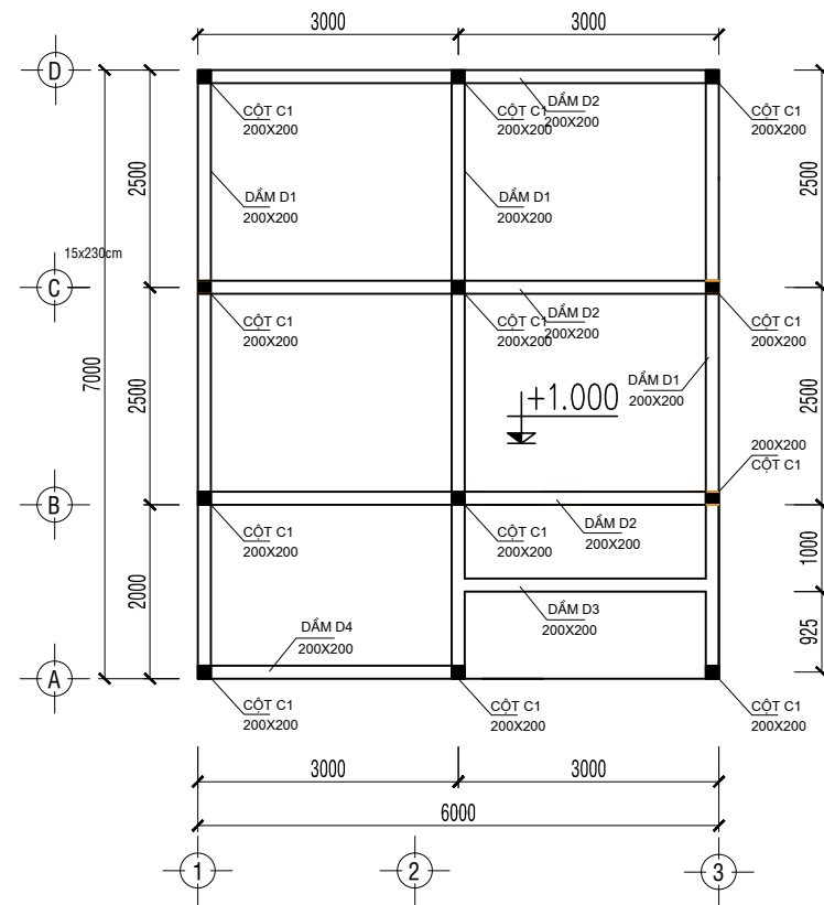
MẶT BẰNG CỘT, DẦM COS +0,9 TL 1/100
