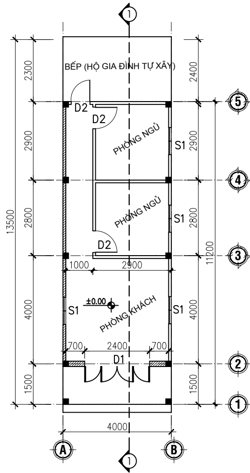
MẶT BẰNG TRỆT
