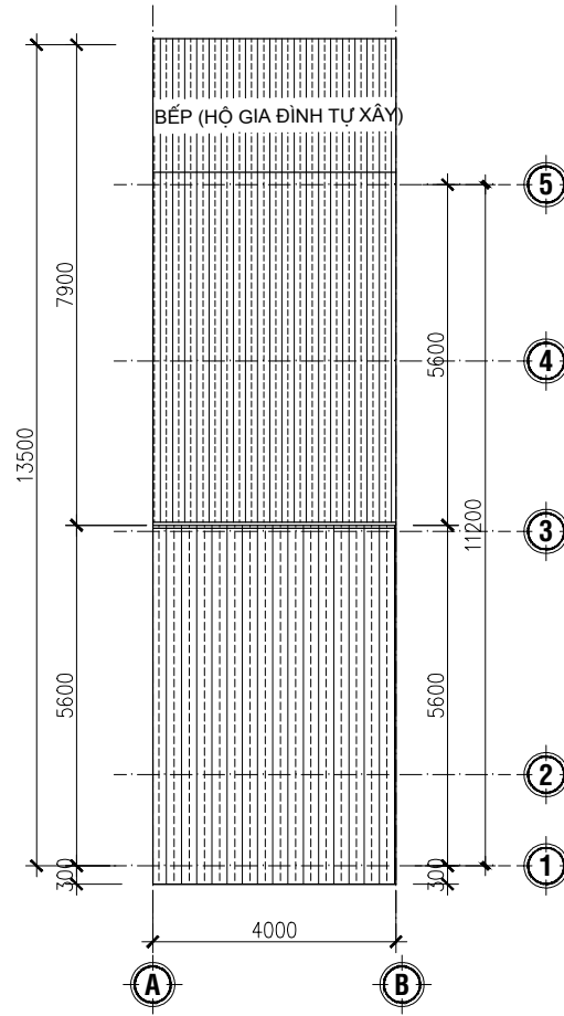
MẶT BẰNG MÁI
