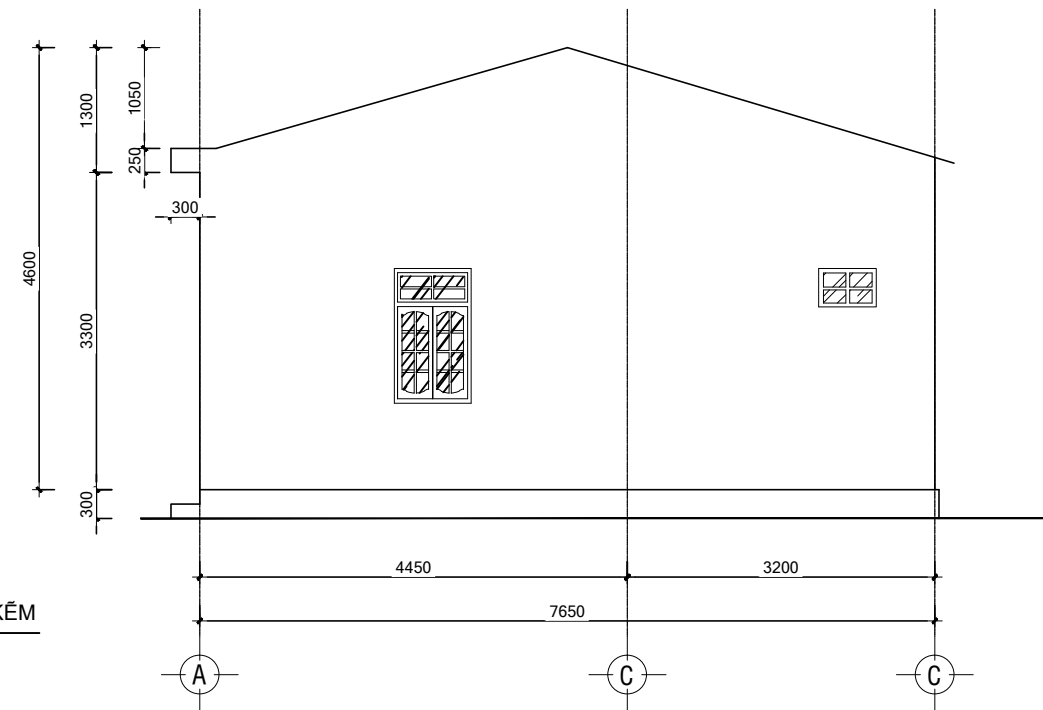
MẶT ĐỨNG BÊN
