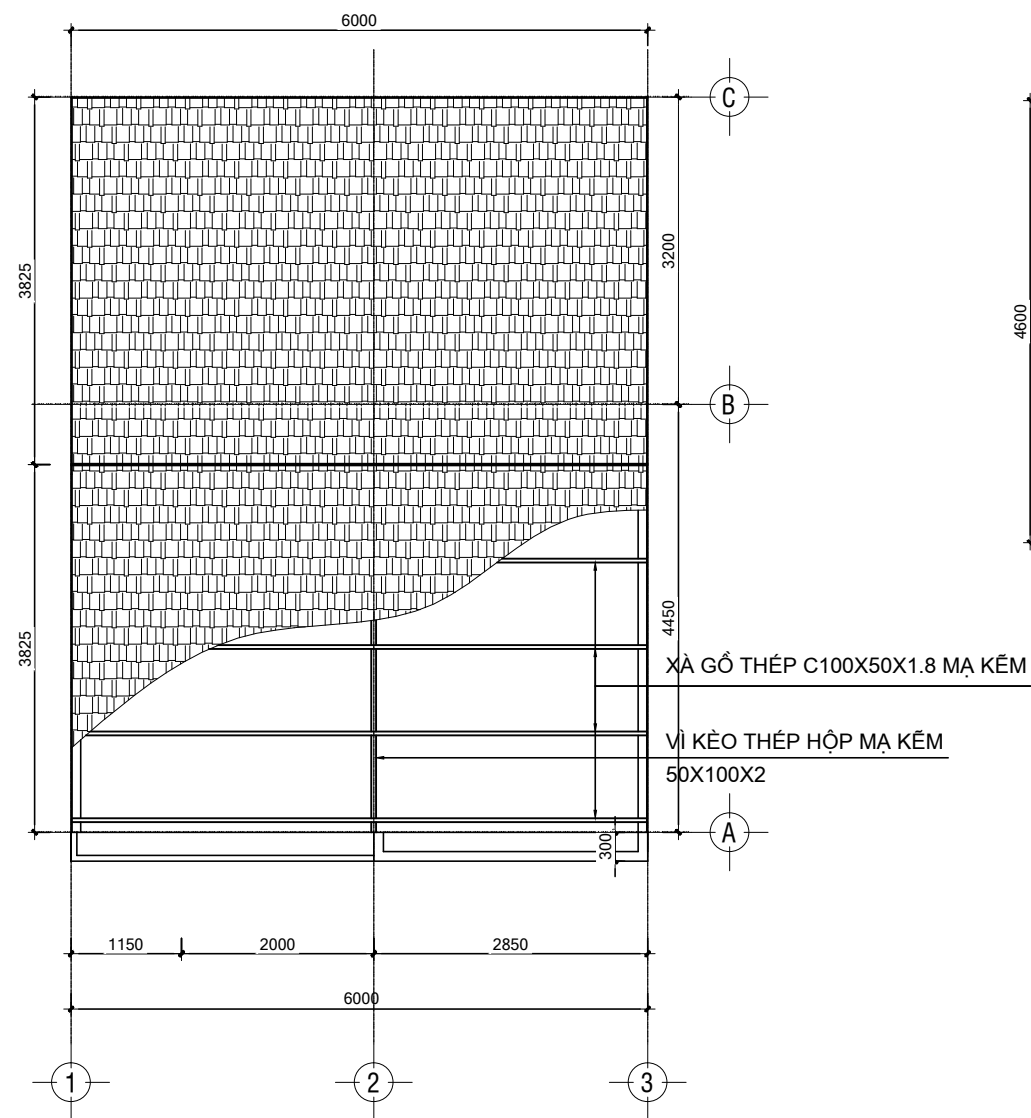
MẶT BẰNG MÁI
