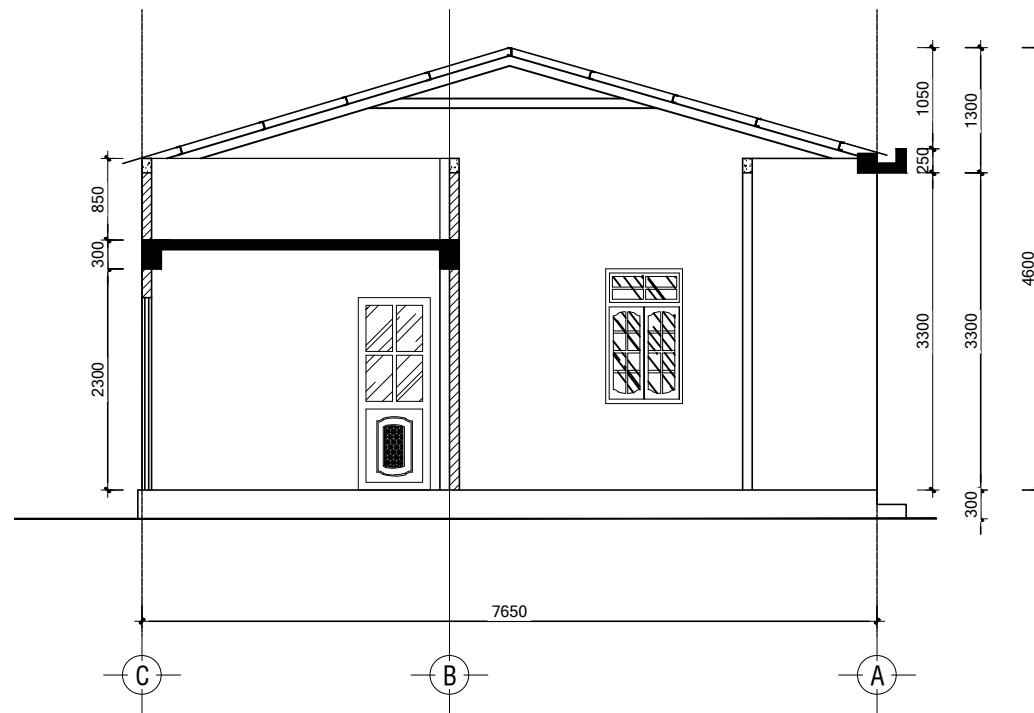
MẶT CẮT 1-1
