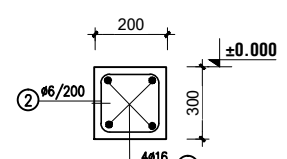
GIẺNG MÓNG DM5 SL: 01CK
