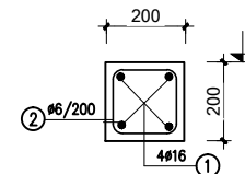
GIẺNG MÓNG DM1 SL: 02CK
