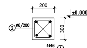
GIẺNG MÓNG DM4 SL: 01CK
