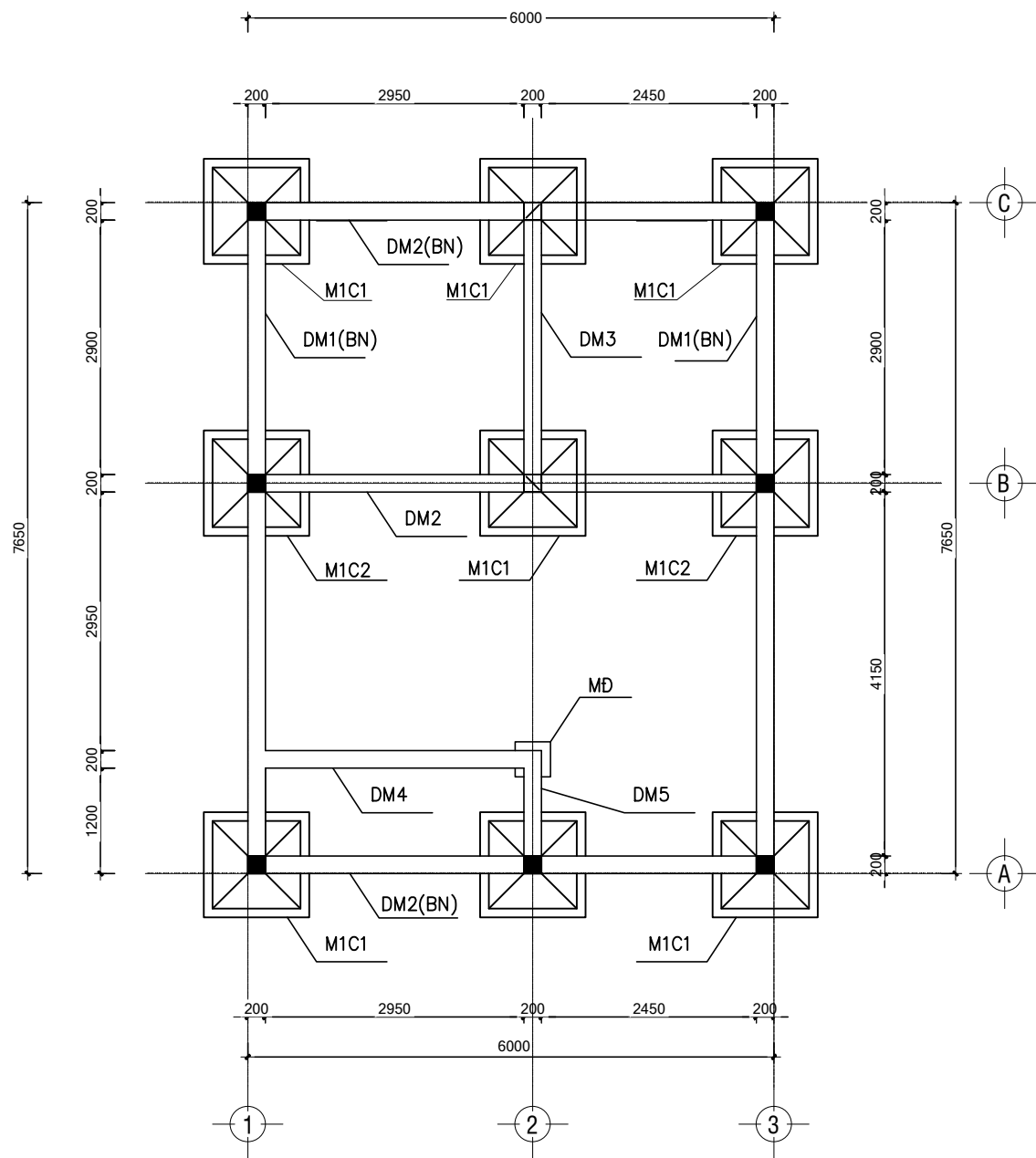
MẶT BẰNG MÓNG M1C1, DM1 TL 1/100
