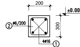
GIẺNG MÓNG DM2 SL: 03CK
